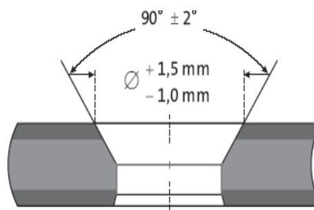
Obr. 5: Tolerance zapuštěné díry
