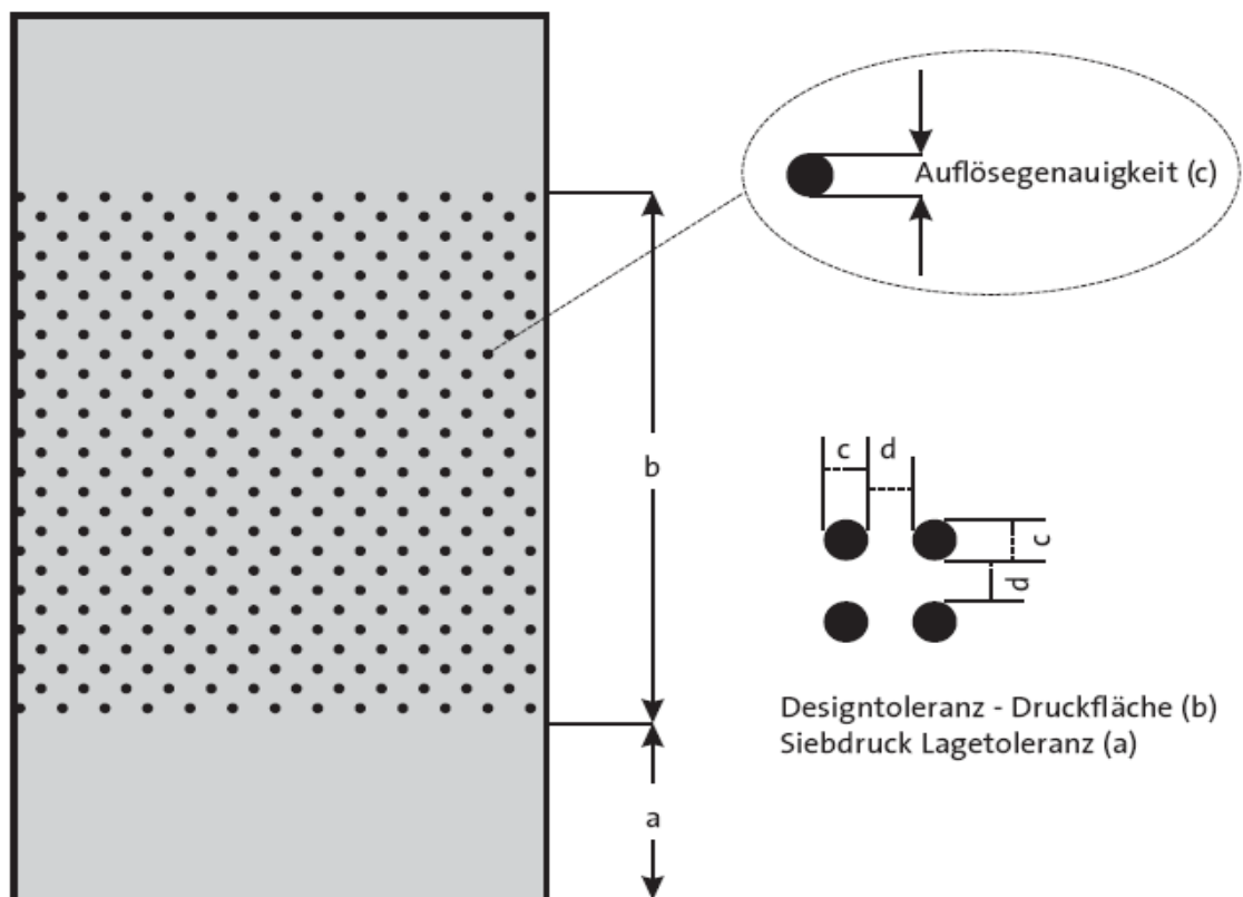
Obr. 10 k tab. 20: Druhy vad/tolerance pro skla se síťotiskem
